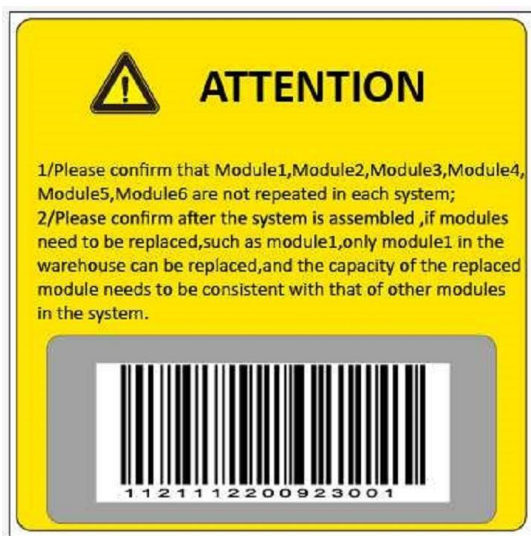
Obrázek 1-2 Štítek bateriového modulu
